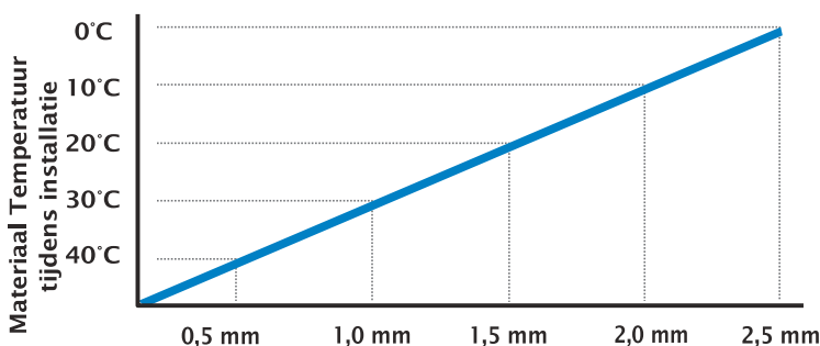
Minimale stuikruimte per lineaire meter
