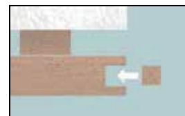
Sluit de uiteinden met een eindplaat (het vooraf frezen van een groef is vereist).
